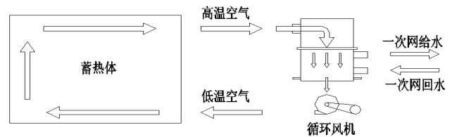
图 2 固体蓄热锅炉供热工作示意图
