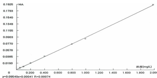
图 1 氨氮气相分子吸收光谱仪分析法标准曲线
