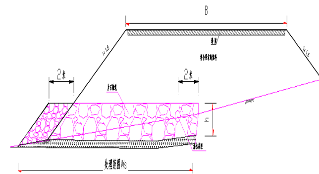
图 4 K150+425 ~ K150+450 段左侧涎流冰治理填石方案图及后期效果预期图
