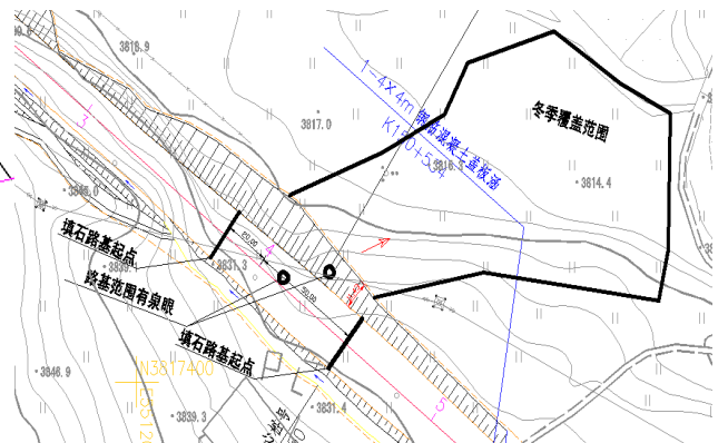
图 4 K150+425 ~ K150+450 段左侧涎流冰治理填石方案图及后期效果预期图
