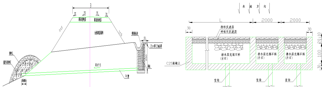
图 1 渗池示意图
