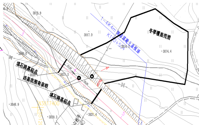
图 4 K150+425 ~ K150+450 段左侧涎流冰治理填石方案图及后期效果预期图
