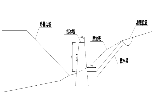
图 3 K149+880 截冰渠横断面示意图
