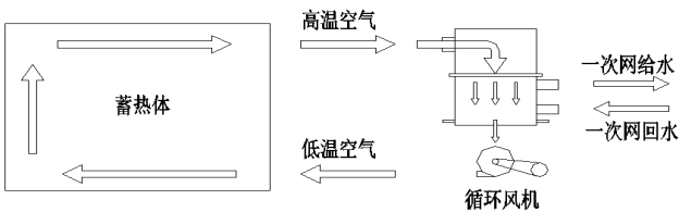
图 2 固体蓄热锅炉供热工作示意图
