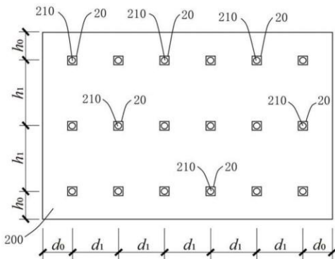
图 2 大体积混凝土基础的状态的示意图，其中可充气弹性气囊未抽出
