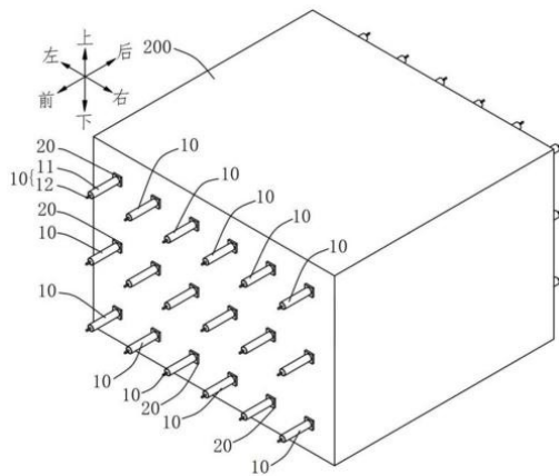
图 1 大体积混凝土基础的状态示意图
