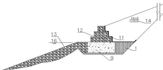
图 4 堤防边坡加固后的断面图
