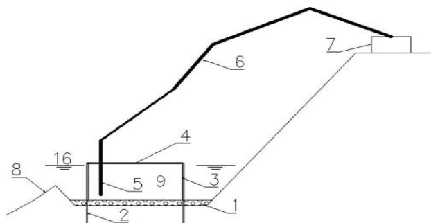
图 1 本方法的施工方案示意图
