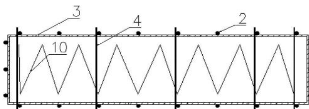
图 2 模板安装固定俯视图
