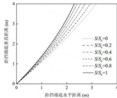
图 2 挡土墙在不同位移时墙后土体潜在破裂面示意图
