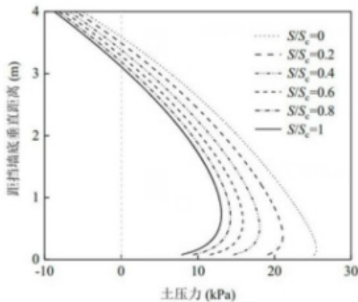
图 3 挡土墙在不同位移时的土压力分布示意图
