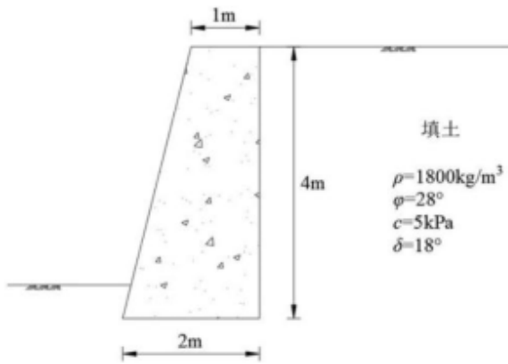
图 1 挡土墙几何参数及土体物理力学参数示意图
