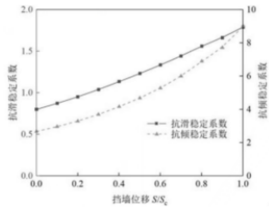
图 4 挡土墙稳定性随挡土墙位移的变化关系示意图
