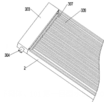
图 5 铺设板、水路管视图
