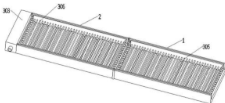
图 4 第一结构强筋、第二结构强筋视图
