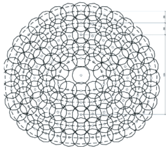
图 1 注浆加固断面设计
