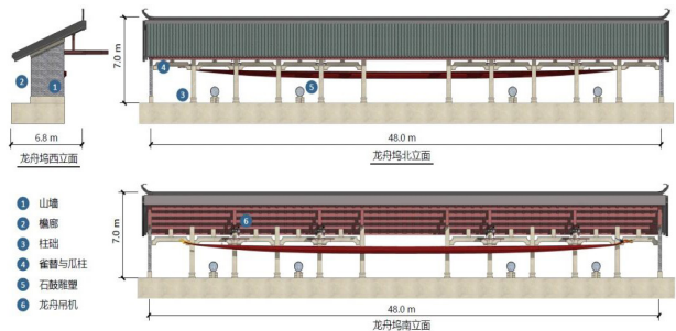
图4 龙舟坞立面图
