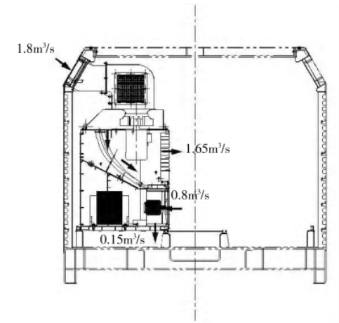
图 8 辅助变压器柜通风支路
