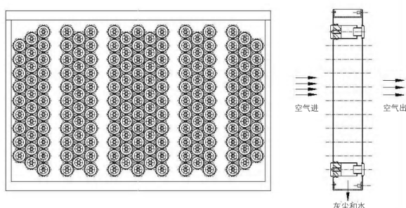
图 14 旋风除尘器
