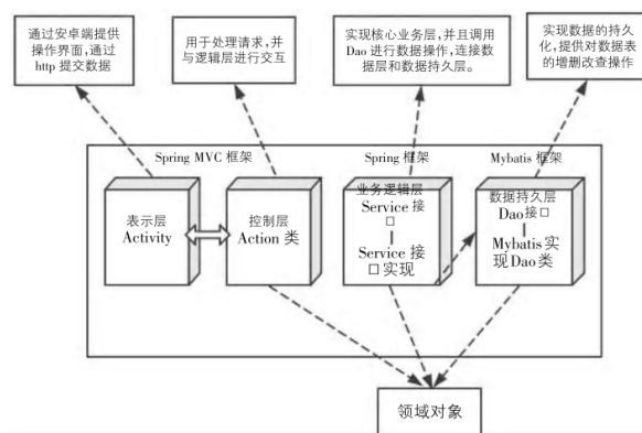
图 2 后端服务架构图
